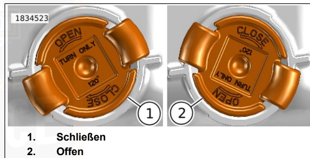
Abbildung 123. Ausrichtung der Ablassschraube
