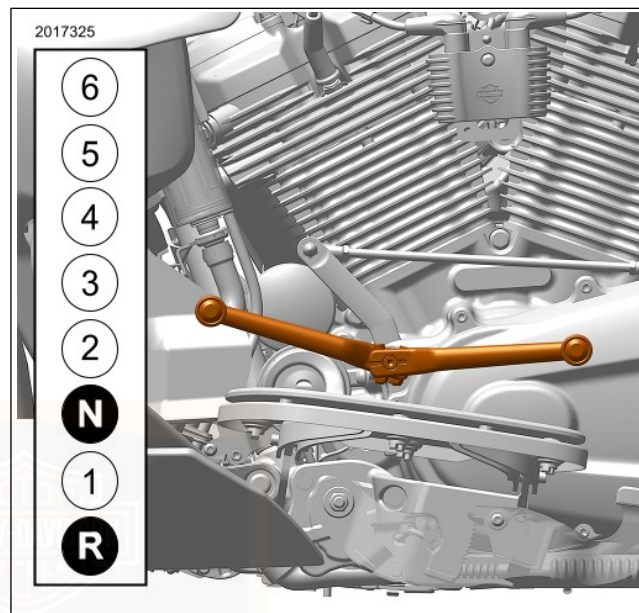
Abbildung 28. Gangschalthebel und Schaltmuster
