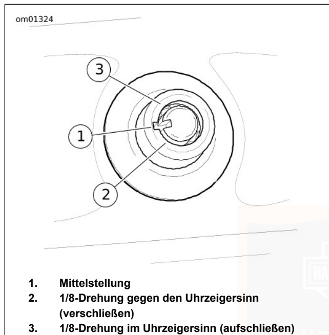
Abbildung 90. Aufbewahrungskofferschloss (Heckklappe)
