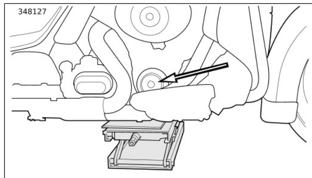
Abbildung 113. Platzierung des Wagenhebers zum Anheben der Vorderradführung
