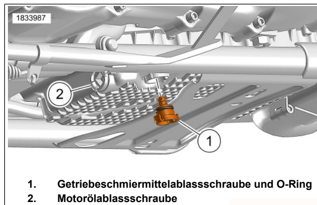
Abbildung 124. Getriebschmiermittelablassschraube PRIMÄRKETTENGEGHÄUSESCHMIERUNG: SYNTHETISCHES ÖL
