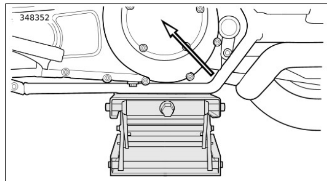
Abbildung 114. Platzierung des Wagenhebers zum Anheben des Hecks
