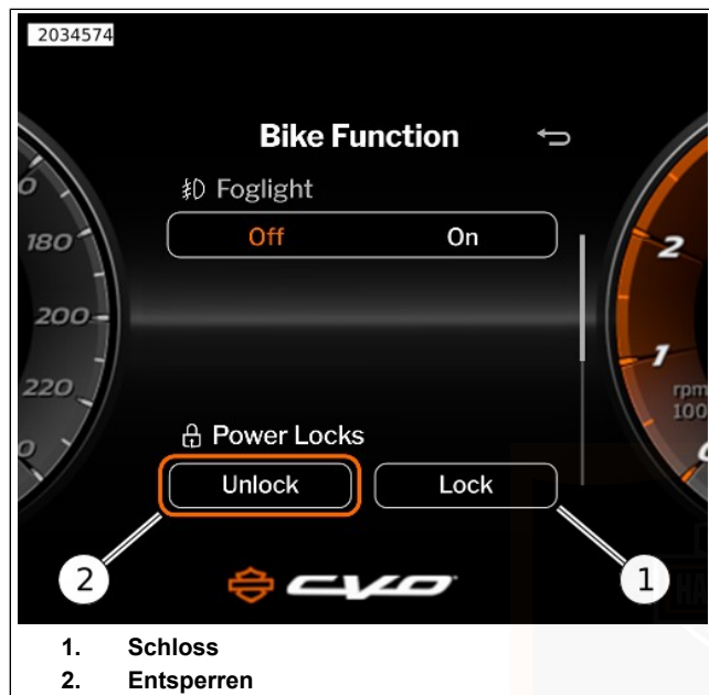
Abbildung 56. Zentralverriegelungen (IFCU)
