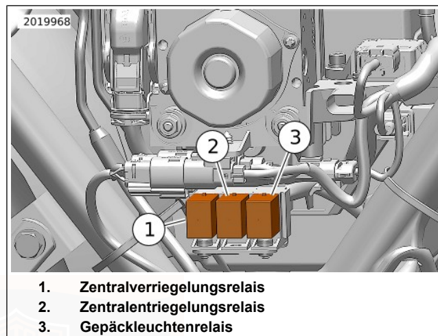
Abbildung 147. Zentralverriegelungsrelais (unter der rechten Seitenabdeckung)
