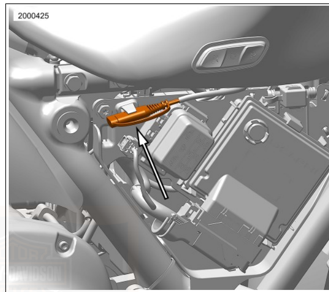
Abbildung 129. Batterieladegerät-Steckverbinder (unter linker Seitenabdeckung)
