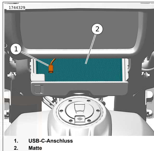
Abbildung 64. Medienfach (offen)
