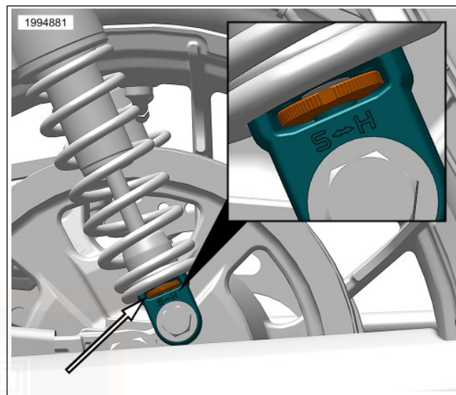
Abbildung 16. Rändelrad der Dämpfungseinstellung (beide Stoßdämpfer)
