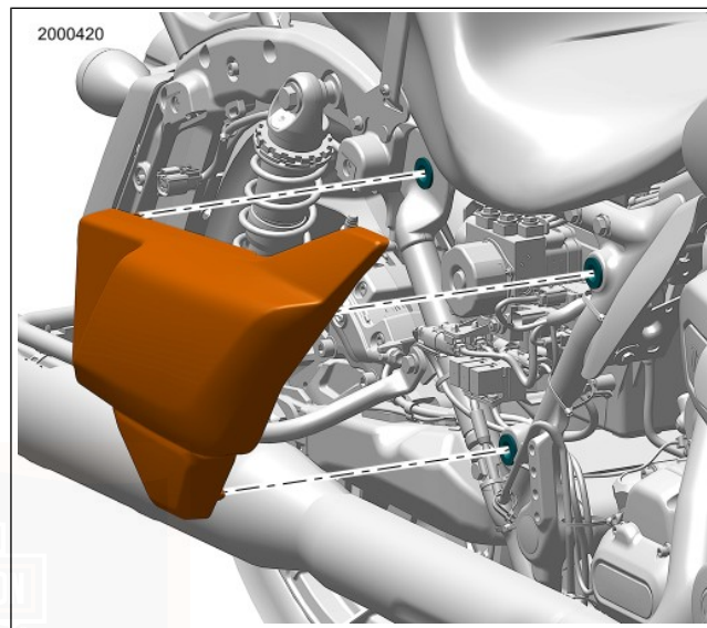
Abbildung 128. Seitenabdeckung BATTERIELADEGERÄT-STECKVERBINDER
