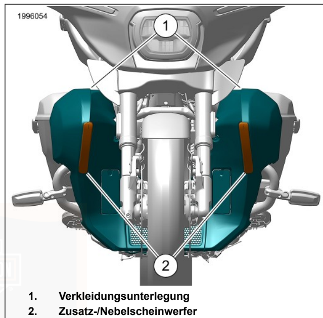
Abbildung 54. Zusatz-/Nebelscheinwerfer ZENTRALVERRIEGELUNGEN
