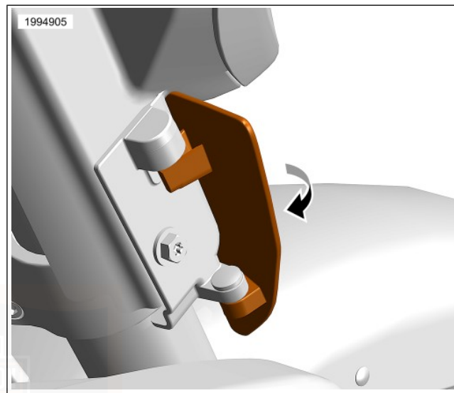
Abbildung 77. Windabweiser: Gabelmontierte Verkleidung UNTERE VERKLEIDUNGEN
