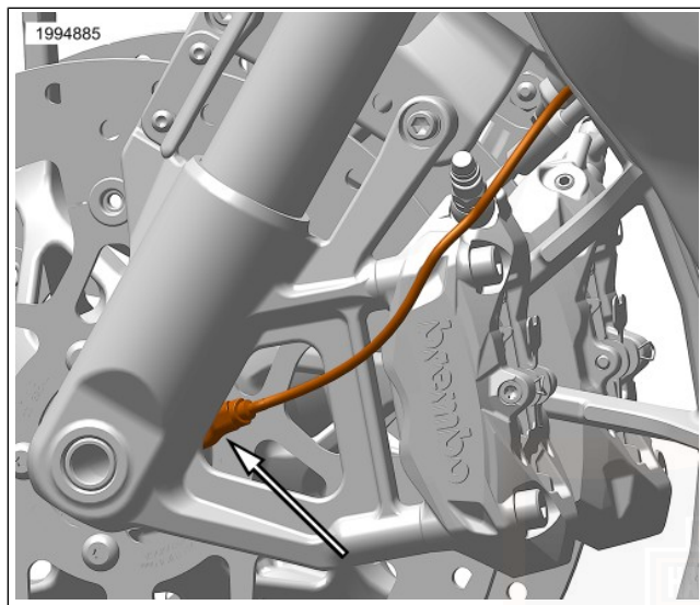
Abbildung 10. Raddrehzahlsensor, (ABS-Identifizierung, typisch)
