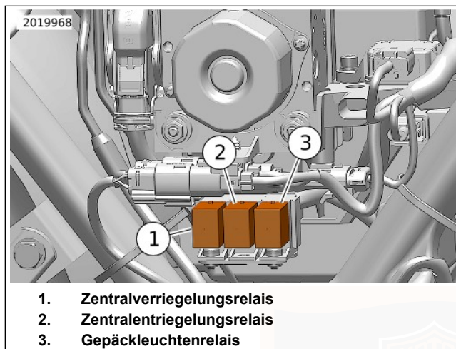
Abbildung 137. Zentralverriegelungsrelais (unter der rechten Seitenabdeckung)
