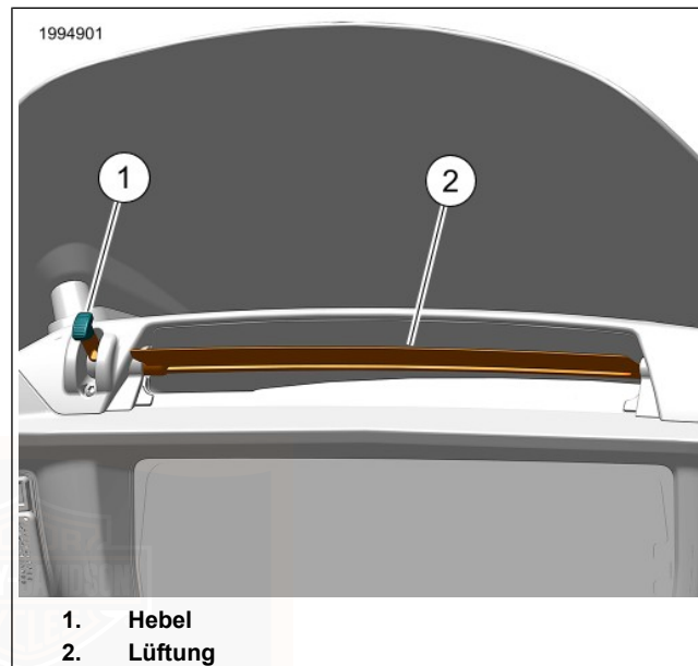
Abbildung 76. Splitstream Verkleidungslüftungsdüse VERSTELLBARE WINDABWEISER
