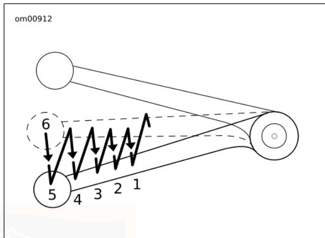
Abbildung 69. Schaltfolge: Herunterschalten FERSEN-/FUßSPITZENSCHALTHEBEL
