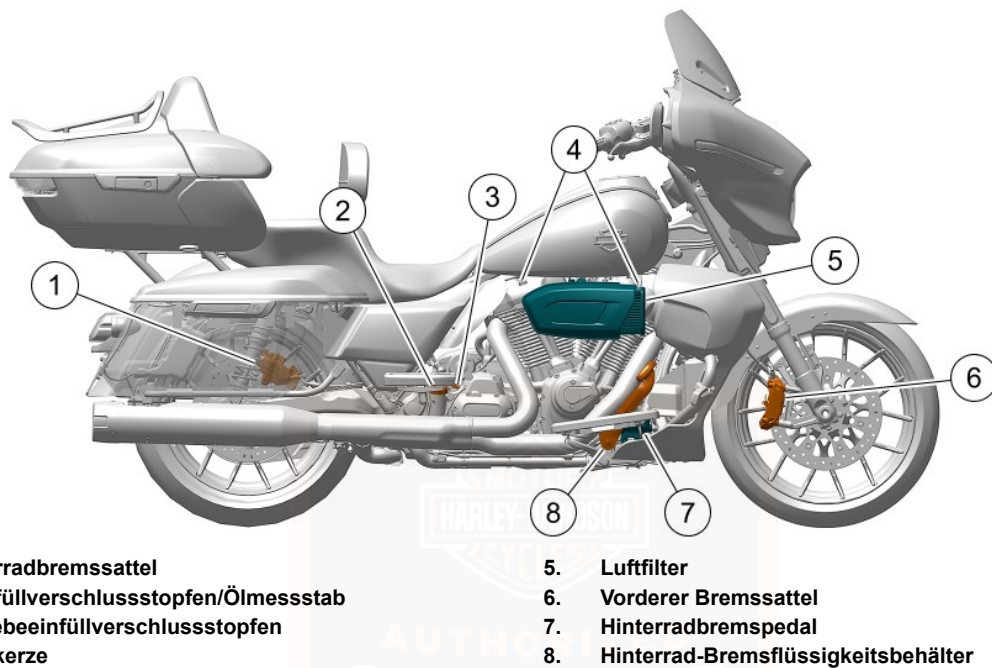
Abbildung 5. Bedienelemente und Servicekomponenten
