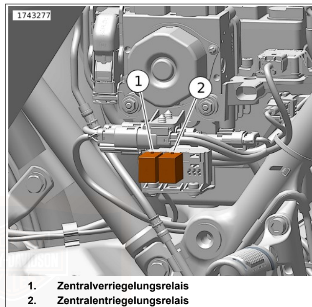
Abbildung 122. Zentralverriegelungsrelais (unter der rechten Seitenabdeckung)
