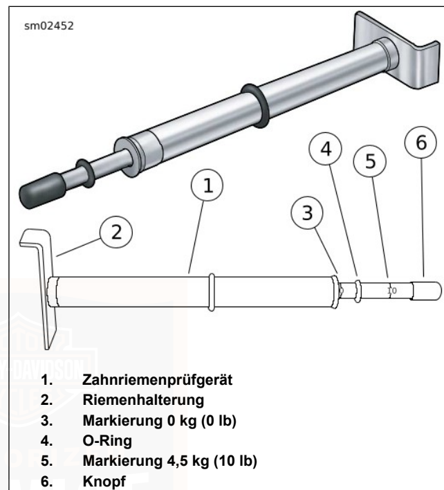
Abbildung 107. Zahnriemenprüfgerät
