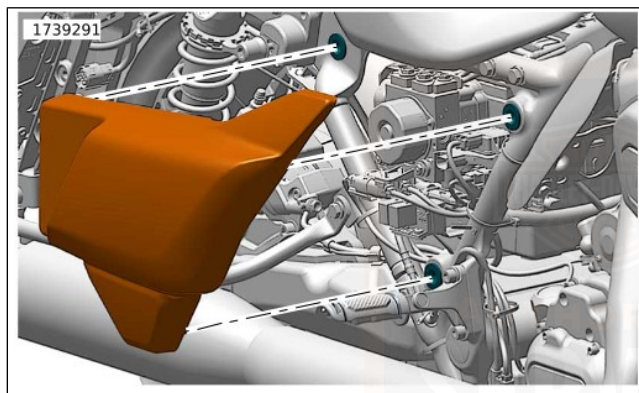
Abbildung 113. Seitenabdeckung
