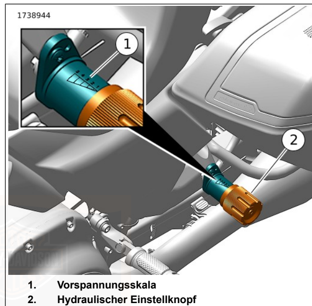
Abbildung 15. Hydraulischer Vorspannungseinstellknopf (linker Stoßdämpfer)
