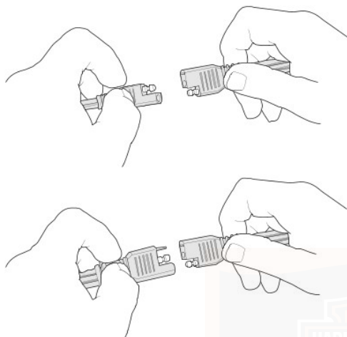
Abbildung 115. Batterieladegerät-Anschluss
