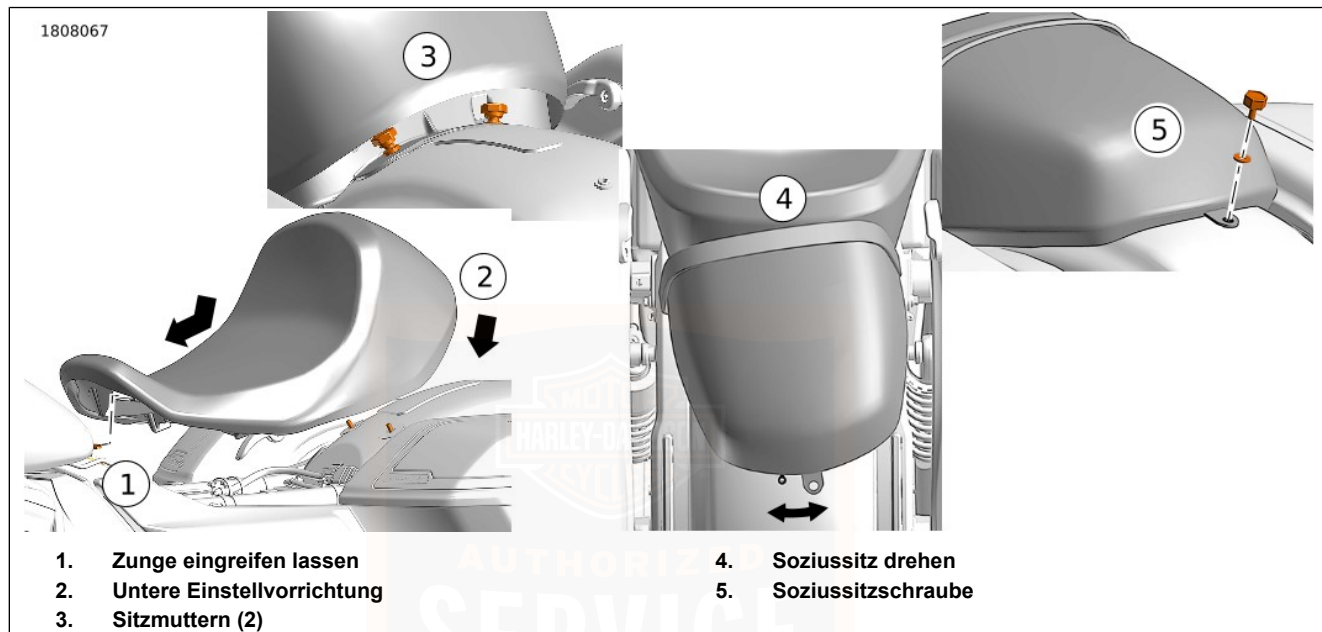
Abbildung 126. Fahrer- und Soziussitz
