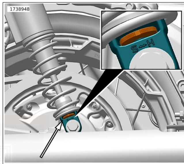
Abbildung 16. Rändelrad der Dämpfungseinstellung (beide Stoßdämpfer)
