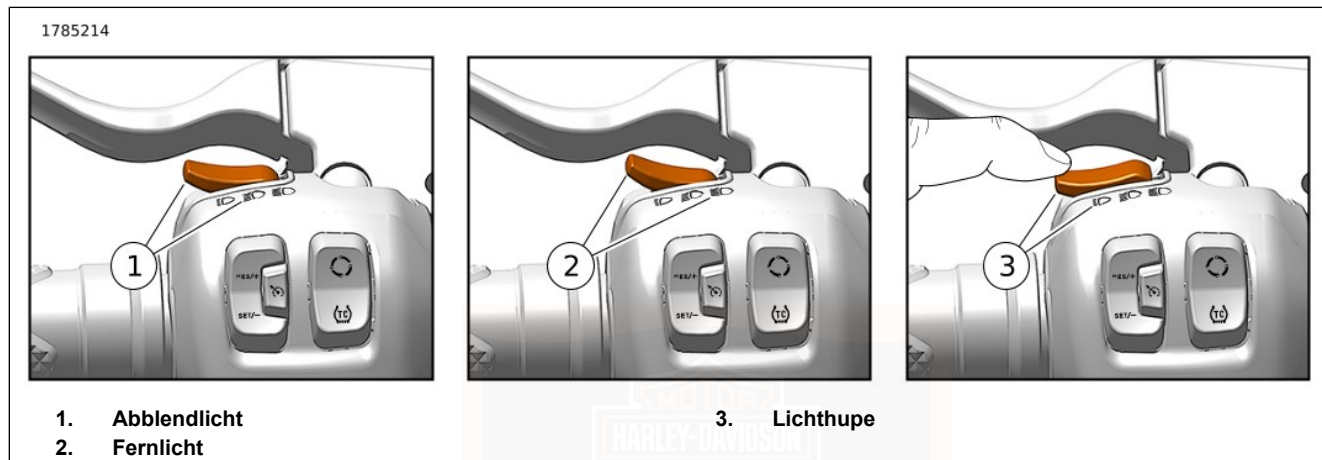
Abbildung 31. Scheinwerferschalter
